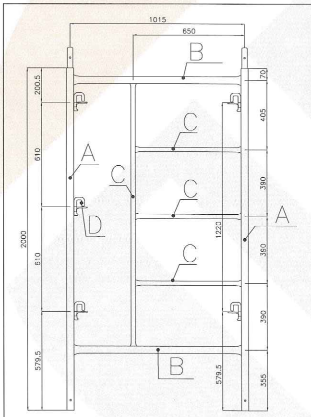
Soldadura del montante con los horizontales en el modelo reforzado
