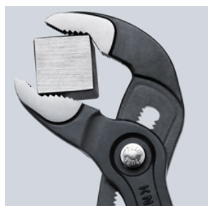
Los dientes desplazados con respecto al sentido de giro provocan un efecto de auto-retención y evitan el deslizamiento sobre la pieza.
