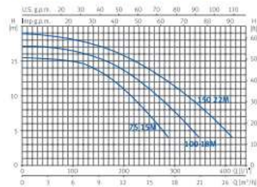
Curvas de funcionamiento a 2900 rpm
