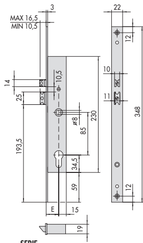
SERIE 16205, 16605 E = 25 - 30 - 35
